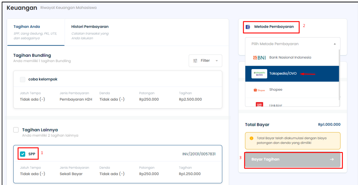
Gambar 2-2 Halaman Proses Generate VA Tagihan Kuliah
